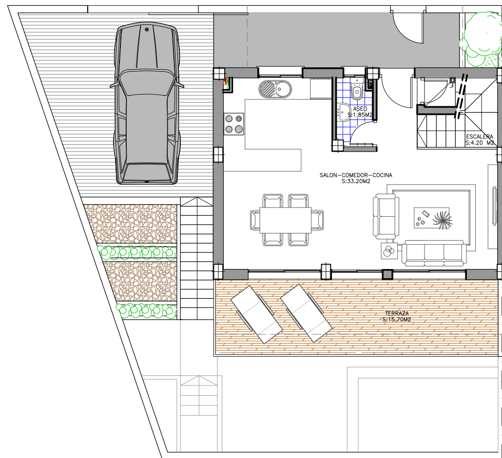
Planta Alta SUP. CONST.: 45.64m 2
