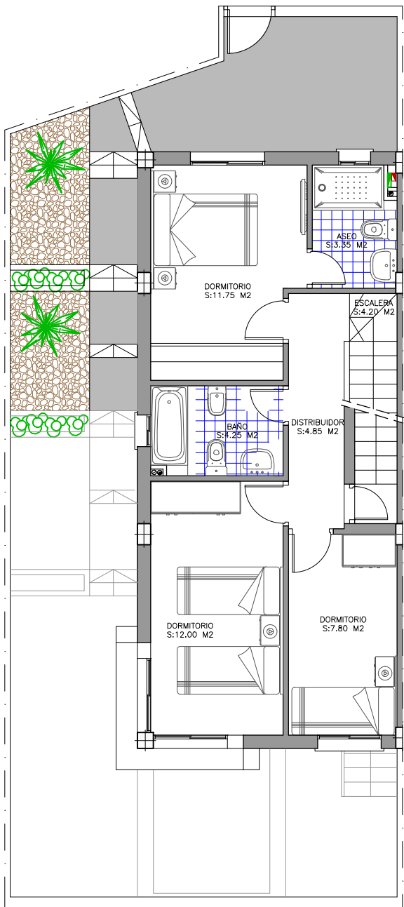
Planta Alta SUP. CONST.: 56.25m 2
